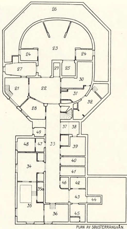
PLAN AV SOUSTERRÄNGVÅN.
