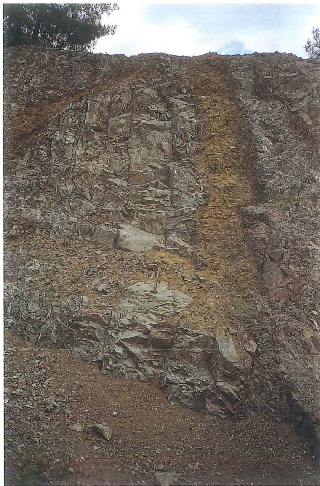
Figur 9. Sværm af stejltstående doleritiske gang intrusioner fra lagserien med gange (gang komplekset). På billedet kan det svagt erkendes, at gangene har en ensidig afkølingskontakt mod venstre, svarende til bort fra spredningsaksen. Gangen i midten med den brune forvitningsfarve er en lidt senere konform intrusion, der har en lidt afvigende sammensætning. Hammerskiftet er 38 cm.
