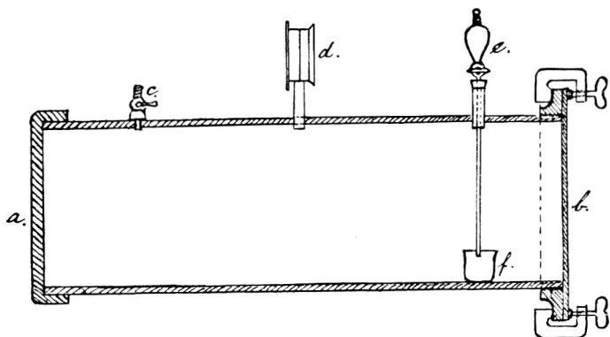
Snit gennem Rygekammeret: a Jærnhætte; b Messingplade, fastgjort med Skruekramper; c Hane til Sugenslangen; d Trykmaaler; e Syrebeholder med Nedløbsrør; f Bæger til Cyanidet.
