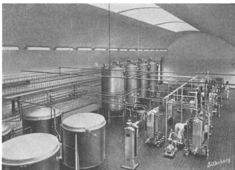
Fig. 2. Interiør fra Mejeriet »Enigheden«, København. Mælketanke og moderne apparater for konsummælken varmebehandling. (Silkeborg Maskinfabrik fot.).
