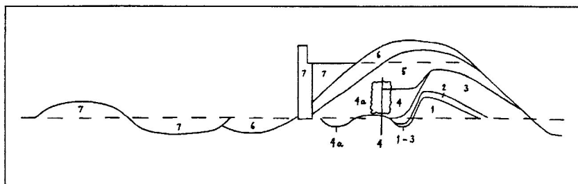
Fig. 5. Danevirkes bygningshistorie som afspejlet i Hovedvolden. Skematisk komposition ved sammenlægning af alle snit. 1 jordvold med lille voldgrav, 7. århundrede. 2 som 1. 3 som 1. 4 palisadevold fra 737, stolpe indkapslet i 4a Kampestensmur med voldgrav. 5 jordvold. 6 jordvold med voldgrav. 7 Valdemarsmuren med voldgrav og forvold, 2. halvdel af 12. årh., øvre del af 5 og 6 sløjfet.
