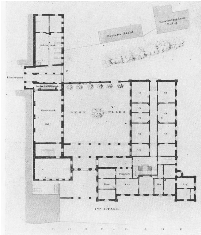
Afb. 17. Stueplan over Skolen i dens endelige Skikkelse.
