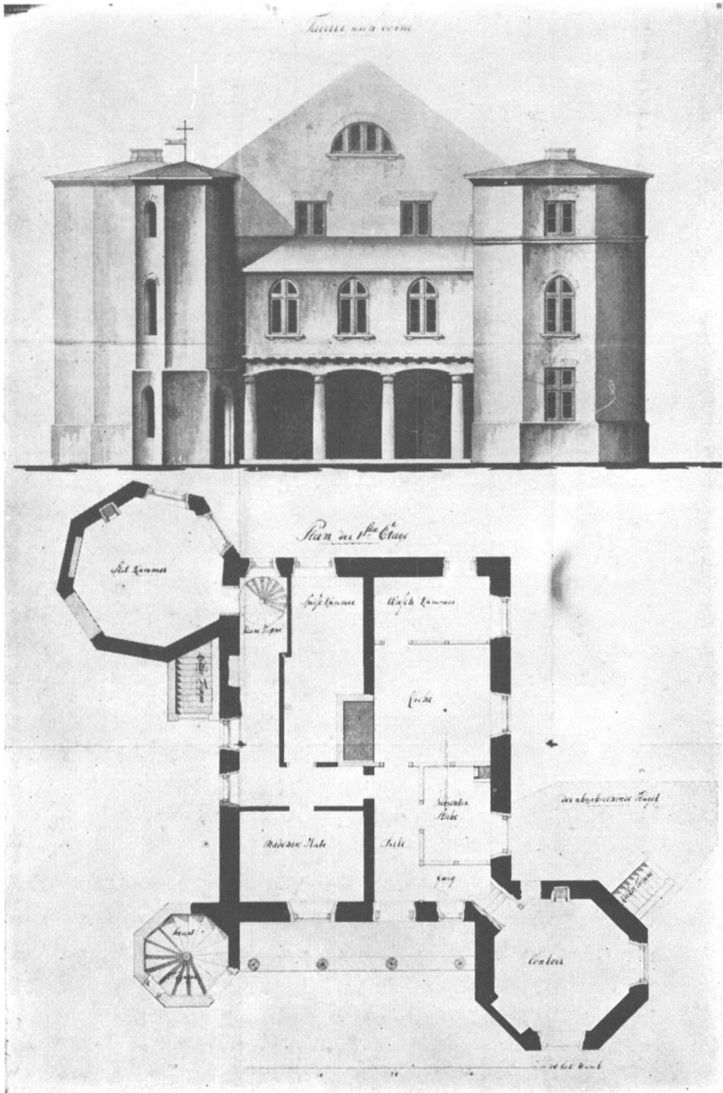
Fig. 5. C. F. Hansens Udkast til det ombyggede Brundlund Slot 1804. Facade, set fra Syd, og Plan over Stuetagen. Farvelagt Tegning i Rigsarkivet.
