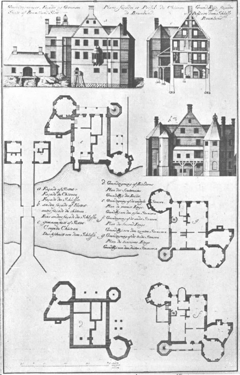
Fig. 4. Facader, Snit og Grundplaner fra Thura: „Den danske Vitruvius“ (1749).
