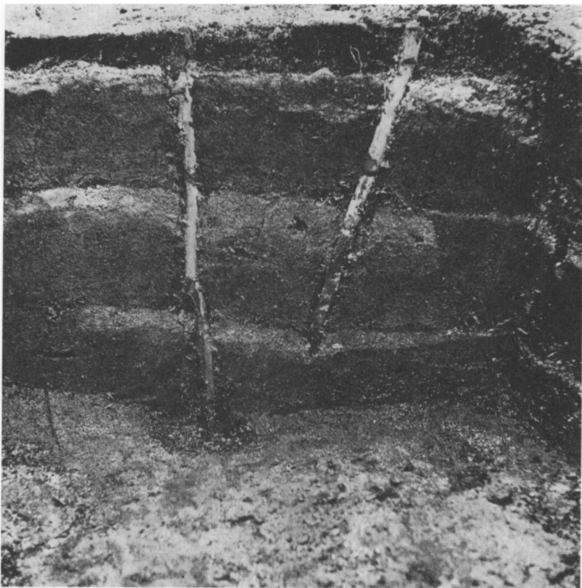
Fig 3. Blokke af tørv har til alle tider været benyttet som byggeemne, men sjældent er det set brugt så konsekvent som i det middelalderlige Solvig. Her ses et snit i tørvevæggen fra det ældste hus på ø nr. 1. Tørvene holdes sammen med lange, spidse træpløkke. Disse to pløkkers længde er ca. 25 og 30 cm.
