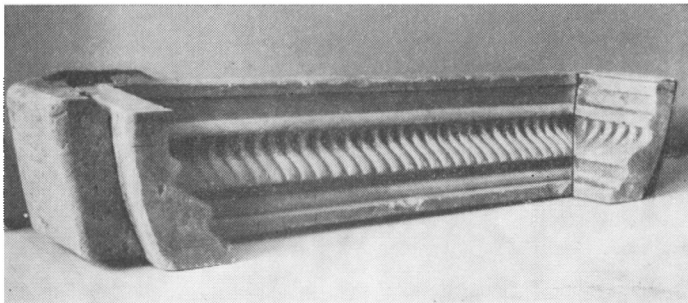
Kakkelform til gesims fra kakkellovnsfabrikken i Christiansfeld. Formen er af gips og har en løs indsats i hver ende. Længde ca. 75 cm. „Den gamle By“, Århus.
