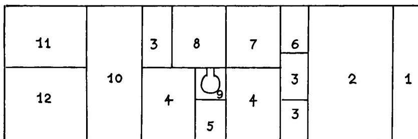
1 = gang, 2 = skolestue, 3 = kamre, 4 = stuer, 5 = forstue, 6 = spisekammer, 7 = køkken, 8 = baggang, 9 = bageovn, 10 = lo, 11 = stald, 12 = lade, (herunder kælder)
