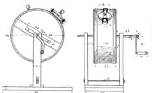
Fig. 12: Svingkærne (2), italiensk/schweizisk model, også kaldet slibestenskerne.
