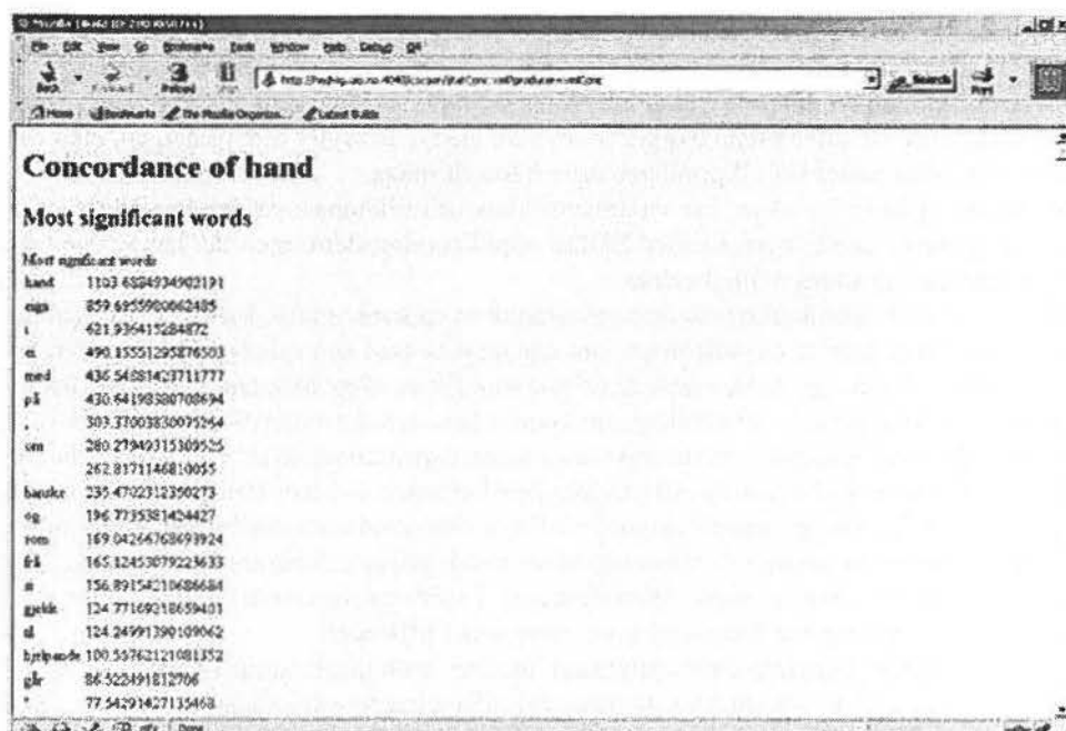
Figur 6: Kollikon försöker att isolera ord som är signifikanta i en kontext med utgångsordet.
