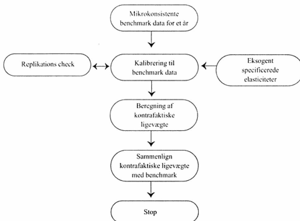
Figur 1. Flowchart ved CGE-modellering.
