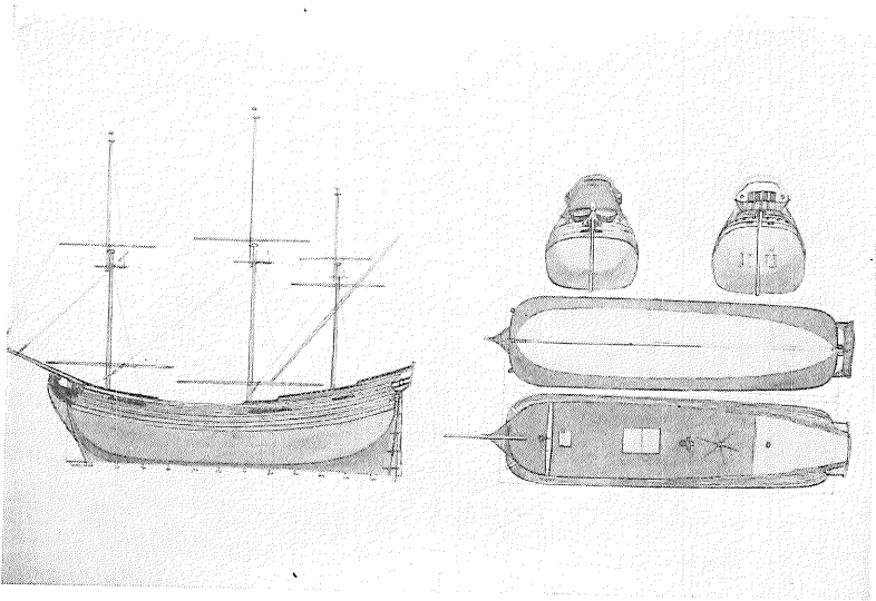
Fløjte med gallerier. Tegning af Adam Silo fra 1700-tallets begyndelse. Tegningen viser fløjten set mod bagbords side (opstalt), mod forstævn, mod agerstævn, mod skrogets bund og mod dæk (dæksplan). Bladets størrelse 55 × 77 cm. Gave fra Handels- og Søfartsmuseets Venner.
