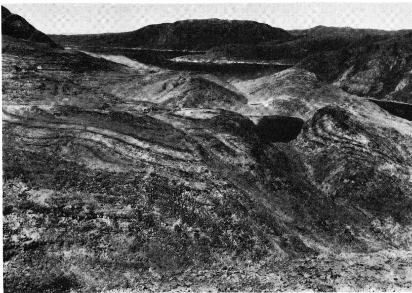
Fig. 26. General view of kakortokites on Kringlerne plateau.
