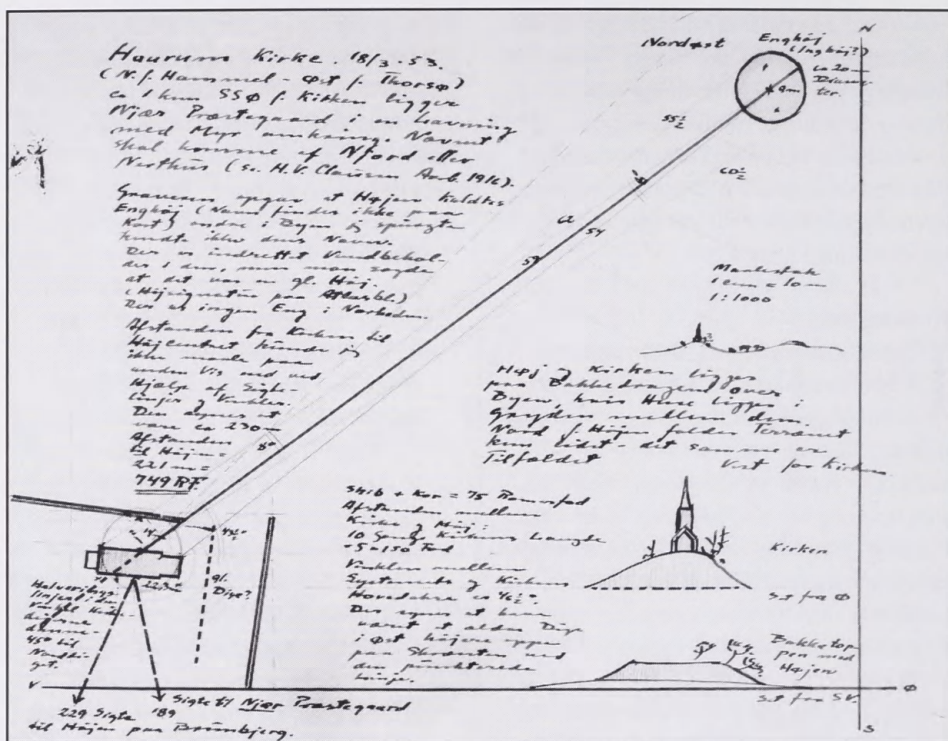
Opmålinger fra Haurum kirke, foretaget af Martin A. Hansen den 18.3.1953.
