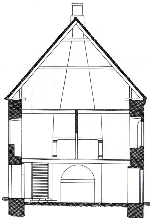
Figur 18. Tværsnit fra 1927 af vestfløjen med skorstenen midt i fløjen. I nedre etage ses køkkenskorstenens forrum og på etagen ovenover den store kamin, som forrummet bærer. Stolpen foran kaminen er fra en tid, da kaminen ikke længere blev brugt. Østfløjen, facader og snit, Bjørnsholm. Antikvarisk-Topografisk Arkiv, Nationalmuseet.
