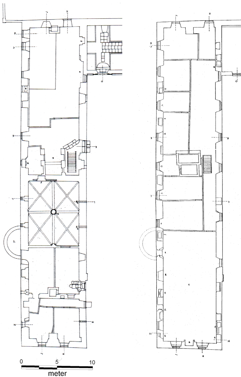
Figur 14. Plan af vestfløjens første og anden etage, 1926. Udsnit af Bjørnsholm, Plan af 1. Stokværk og Bjørnsholm, Plan af 2. Stokværk. Antikvarisk-Topografisk Arkiv, Nationalmuseet.
