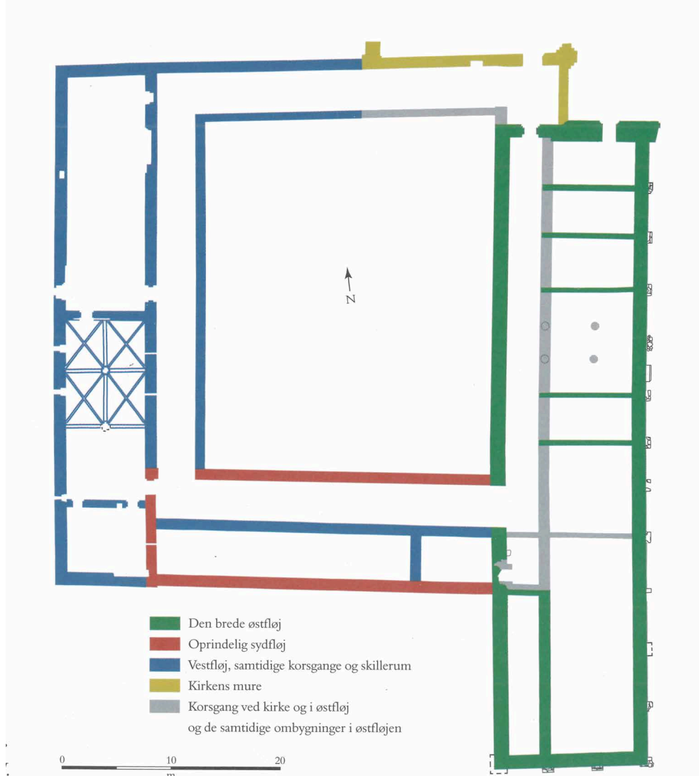
Figur 3. Grundplan for Vitskøl Klosters centrale klosteranlæg umiddelbart før Reformationen i 1536. Efter Hjermind og Støttrup Jensen 2016.
