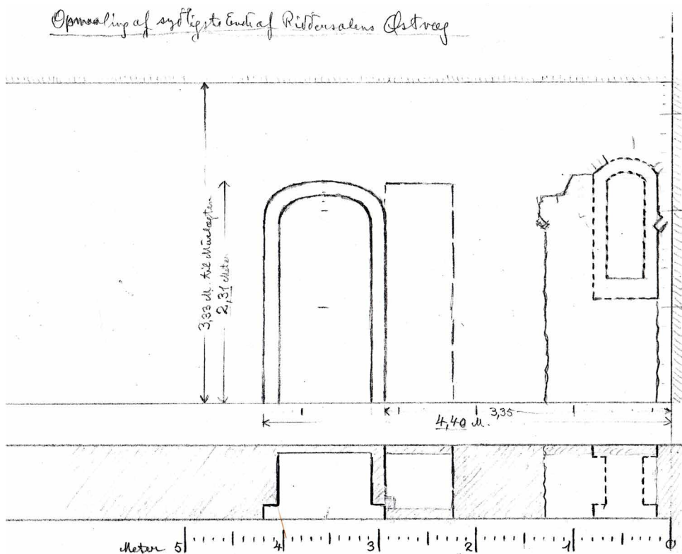
Figur 17. Opmåling af fruerstuens østre murens sydligste ende. Et rekonstrueret fladbuet sengotisk vindue (jf. figur 4) i østmuren er øjensynligt udvidet til et større vindue, som det store kurvehanksbuede vindue ved siden af. Rester af et fladbuet stik viser, at der senere i vinduet er indsat en lavere døråbning, der førte ud til den karnap, som blev opført i 1574. C.M. Smidt 1927: Opmaaling af sydligste Ende af Riddersalens Østvæg . Antikvarisk-Topografisk Arkiv, Nationalmuseet.
