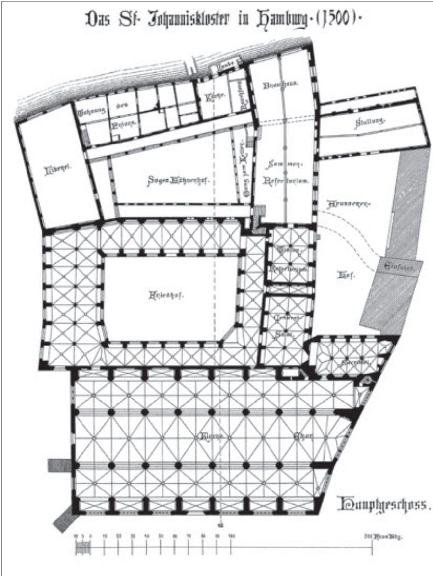
Fig. 31. Grundplan af dominikanerklosteret i Hamburg. Den store treskibede kirke med kapelrækker mellem stræbepillerne blev genopført efter en brand i 1424. Korets skrå afslutning skyldes, at kirken blev bygget helt ud til gaden Hinter dem Breitengiebel. Vestfløjen og dele af korsgangen var nok fra samme tid som kirken, mens andre dele af klosteret blev opført i 1300-tallet. – Efter Først 2014.
