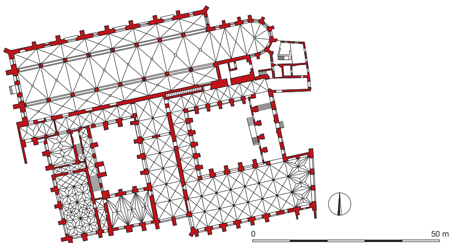
Fig. 10. Grundplan af dominikanerklostret i Stralsund. Koret blev opført i 1282, mens skibet dateres til 1292 og 1308. Klosterbygningerne repræsenterer mange byggefaser fra 1200-tallet til o. 1500. Den store treskibede sal i sydøst fra tiden o. 1420 opfattes som klostrets sommerrefektorium, Remter. De to klostergårde med korsgange skal muligvis ses i problematikken omkring offentlige og lukkede fratergårde. – Tegning: Martin Ebert, efter Ebert & Grundner 2009.
