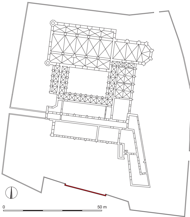
Fig. 20. Rekonstrueret plan af franciskanerklostret i Wismar. Kirken har haft den typiske nordtyske form som en treskibet hallekirke med et langstrakt kor. Det antages, at det søndre sideskib har været delt i to stokværk, således at korsgangen ind mod kirken har forløbet i sideskibets nederste stokværk. – Tegning: Martin Ebert, efter Ebert & Grundner 2009.
