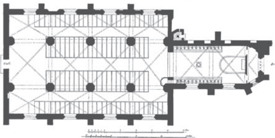
Fig. 40. Grundplan af klosterkirken i Fåborg. Kirken, der hører til den seneste del af middelalderen og derfor ikke blev helt færdig før Reformationen, har fået den karakteristiske planløsning, som kendetegner de betydeligt ældre tiggerklosterkirker i Nordtyskland. Dog er skibet ikke en hallekirke, men en pseudobasilika. – Efter Lorenzen 1912
