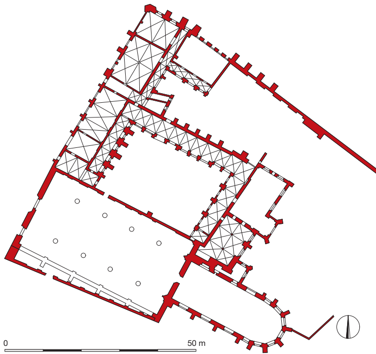
Fig. 11. Grundplan af franciskanerklostret i Stralsund. Kirken blev påbegyndt i anden halvdel af 1200-tallet, og det centrale klosteranlæg regnes for færdiggjort i begyndelsen af 1300-tallet. Også her kom der senere en ekstra klostergård længere væk fra kirken. De to gårde er tolket som henholdsvis en offentlig og en privat gård. – Tegning: Martin Ebert, efter Ebert & Grundner 2009.
