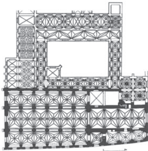
Fig. 37. Grundplan af dominikanerkirken i Danzig og klostergården nærmest kirken. Kirken blev opført i løbet af anden halvdel af 1300-tallet. Karakteristisk for området er der tale om en treskibet hallekirke med et langt etskibet kor. Som brugt i Danzig er hvert af skibene dækket af sit eget saddeltag. Brugen af stjerne- og nethvælv var helt dominerende i senmiddelalderen i Østpreussen og Danzig. – Efter Herrmann og von Winterfeld 2015.
