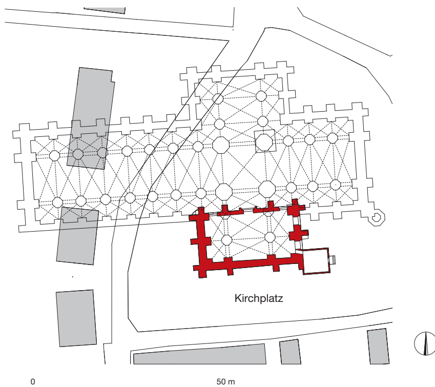
Fig. 17. Rekonstrueret grundplan af klosterkirken i Neuenkamp (Franzburg). Den 90 m lange kirke regnes for opført i perioden 1280-1340. Såvel skib som kor og tværskib var opført som en treskibet hallekirke med stor indvendig højde. – Tegning: Martin Ebert, efter Ebert & Grundner 2009.
