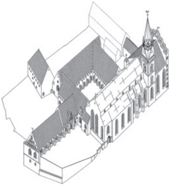
Fig. 34. Isometrisk tegning af Burgkloster i Lübeck set fra sydvest. Klosteranlægget består af bygninger fra forskellig tid. Ældst er nordfløjen, der i substansen er et genbrug af den store sal i Valdemar Sejrs borg fra før klosters oprettelse. Den nu nedrevne kirke indeholdt bygningsdele fra 1200-, 1300- og 1400-tallet. Bygningen mod vest, der er opført på en betydelig opfyldning og underjordiske subkonstruktioner, er klosters såkaldte "Skriftemålsbygning" fra midten af 1300-tallet. – Tegning: M. Gorski, efter Schneider 2014.
