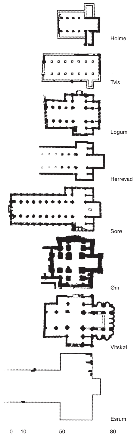
Fig. 39. Grundplaner af danske cistercienserklosterkirker. De fleste kirker fik ikke den tilsigtede længde. Blandt de afbildede planer er det lidt usikkert, om Esrum og Herrevad blev udbygget til fuld længde. Idealet har været en kirke af Fontenay-type, dvs. en treskibet basilika med tværskib, rektantet kor og rektantede kapeller ved tværskibets østside. Kirken i Vitskøl fik ret hurtigt en koromgang med ni apsider, mens munkene i Holme og Tvis med tiden opgav at opføre et tværskib. – Efter Callesen 2011.
