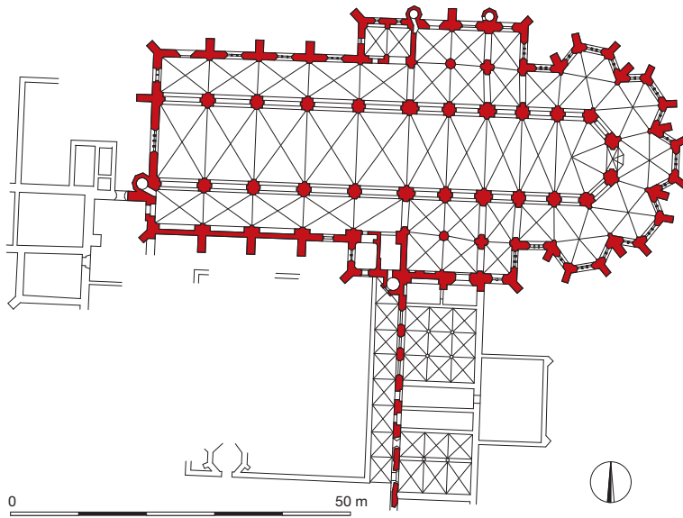
Fig. 29. Grundplan af cistercienserklostret i Doberan. Kirkens planløsning har haft stor betydning for udformningen af hovedkirkerne i København (Vor Frue) og Malmø (Sankt Petri). – Tegning: Martin Ebert, efter Ebert & Grundner 2009.
