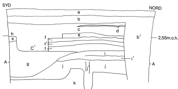
Fig. 4: Nicolaigården. Snit. 1:40. a recent broilægning, b gråsort jord med teglbrokker, b 1 grube, c gråt, humøst sand, c 1 som c, men med mange sten, grube, d gult sand, e gult, let leret sand, f sortgrå humusjord med aske, f 1 som f, men uden aske, g gytjeagtig humusjord med træ, knogler og sten, grube, h rester af broilægning på lag e, udbredt i tilstødende jordvæg, i sortgråt humøst sand med brændte lerrester, i 1 som i, men uden brændte lerrester, j lagdelt, gråt, svagt humøst sand, gruber og stolpehuller i undergrund, j 1 som j, stolpespor, k gult sand, undergrund. Koten A-A angiver normallinje for uforstyrret undergrund.
