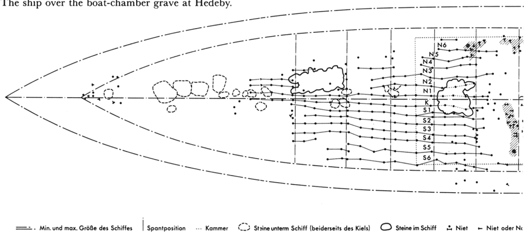
Fig. 2: Skibet over bådkammergraven i Hedeby. (Efter Müller-Wille 1976, Abb. 9).
