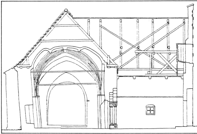
Fig. 4: a: Tostokværksvåbenhuset i Spørring, Aarhus amt. Forf.fot. b: Tværtsnit set fra vest. Linjen over det lille vindue markerer andet stokværks gulvniveau. Opmåling 1953 af A. Skov og F. Beyer 1980. Danmarks Kirker, Aarhus amt. 1:150. c: Oprindeligt vindue på våbenhusets vestside. Forf. fot. a: The two-storied porch in Spørring, Aarhus amt. b: Transverse section, drawn 1953 by A. Skov and F. Beyer 1980. c: Original window in the westwall.
