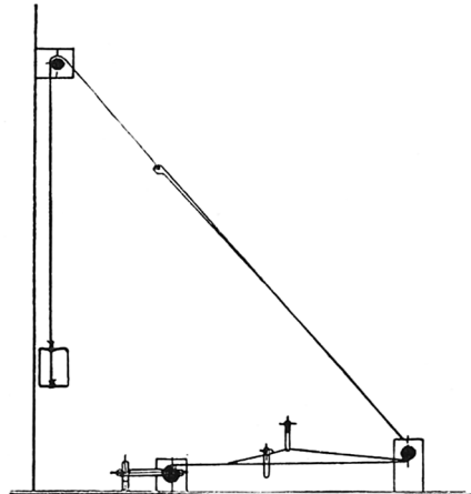
Fig. 12. Diagram visende Vægtens Ophængning bagved Væverens Plads, e. A. Braulik, 1900. Diagram illustrating suspension of the weights behind the weaver's position.
