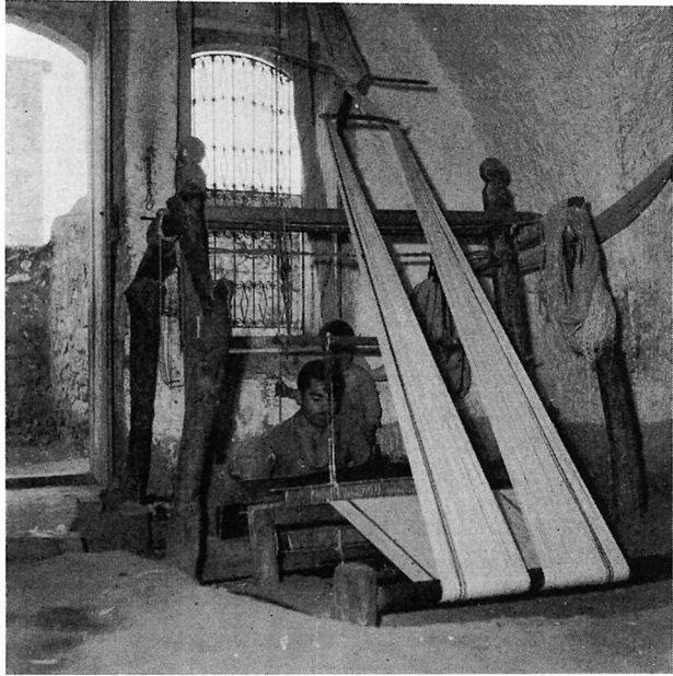
Fig. 6. Vandret Væv med Trædning i Grube. Væven har 8 Stolper. Azaz, Nordsyrien, 1961. M. H. fot.
