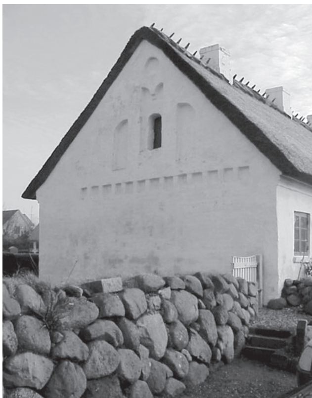
Fig. 12. Vestgavlen på Mesinge kirkelade, Bjerger herred, Odense amt. Bemærk udvidelsen mod nord. – Foto: Mikael Marnø Bjerregaard 2003.
