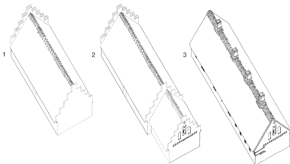
Fig. 5. Bygningshistorien for Mesinge kirkelade, Bjerge herred, Odense amt. 1: kirkeladens oprindelige volumen, 2: kirkeladen efter den i 1589 omtalte vestforlængelse, 3: kirkeladen efter ombygningen i 1822, hvor bygningen i det store og hele fik sit nuværende udseende. – Efter Søndergaard 1979, s. 135.
