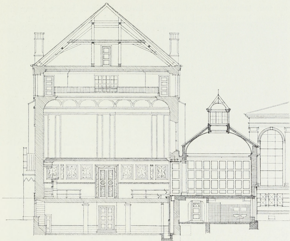
Fig. 1. Tværsnit af Festsalen med den nye Tilbygning.
