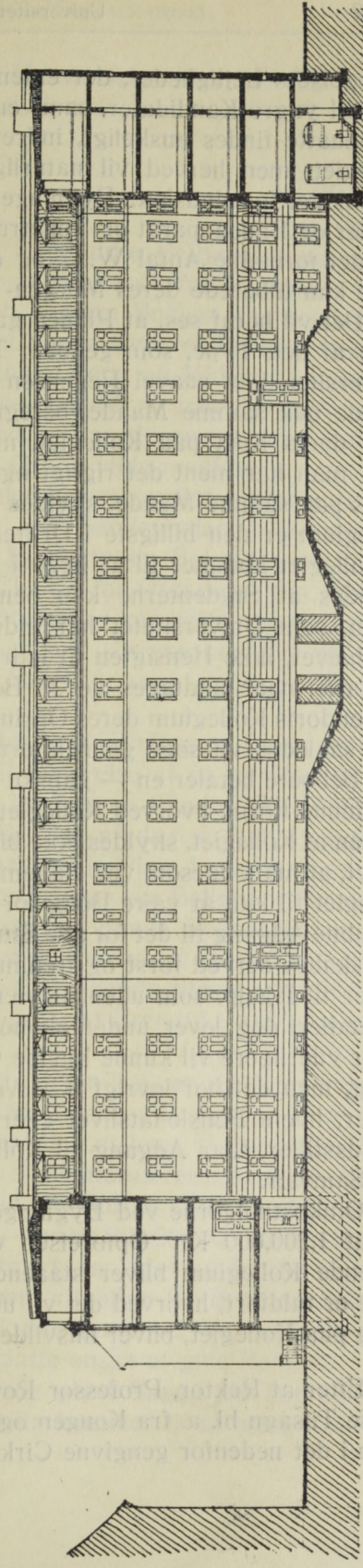
GAARDFAÇADE, MED SNIT AF FOR- OG BAGHUS.
