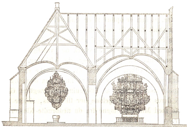
Tværsnit af Præstø Kirke 1:288.
