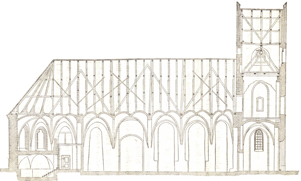
Længdesnit af Præstø Kirke 1 : 288.
