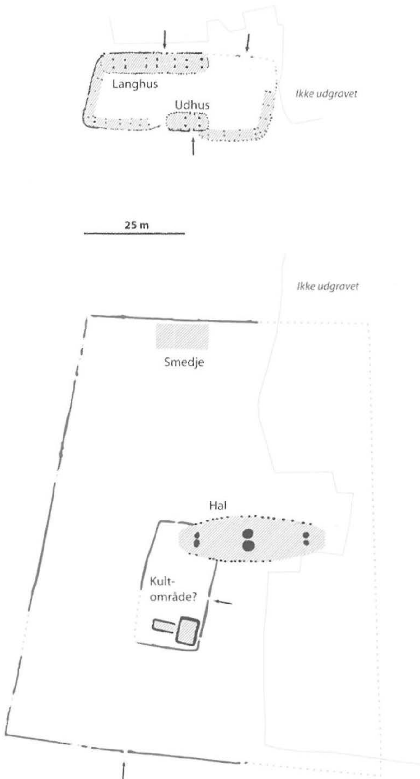
Oversigtsplan over hallen ved Tissø nord for Slagelse (nederst) og gårdsparcel fra Nr. Snede (øverst), der tydeligt viser forskellen i størrelse, både for parcellens areal, men også for de enkelte huses grundplan. Begge planer er fra det 7. årh. (Tissø efter L. Jørgensen (2002) i Plats och Praxis ).
