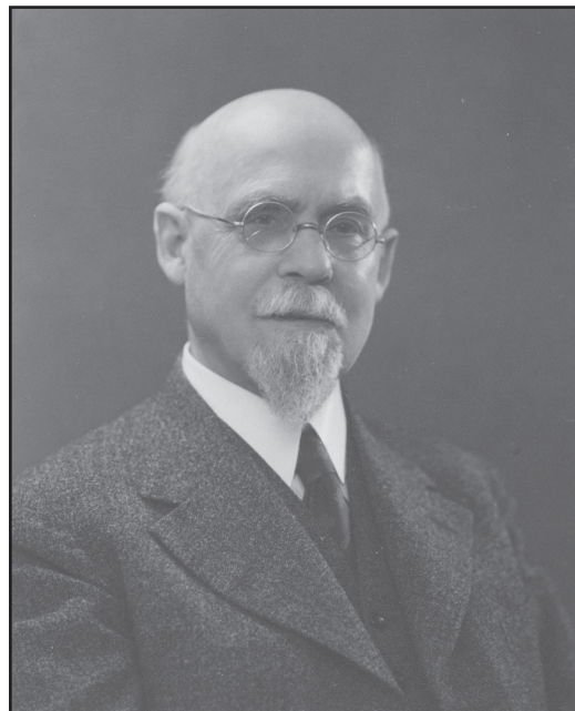
Fig. 1: Aage Friis (1870-1949), professor i historie ved Københavns Universitet fra 1913 til 1935. Hovedvægten i hans livsværk lå i udforskningen af de politiske og kulturelle forbindelser mellem Danmark og Tyskland i 1700-tallet og af det sønderjyske spørgsmål fra 1864 frem til genforeningen i 1920. Foto fra først i 1930'erne: Elfelt & Co, Det Kgl. Bibliotek.
