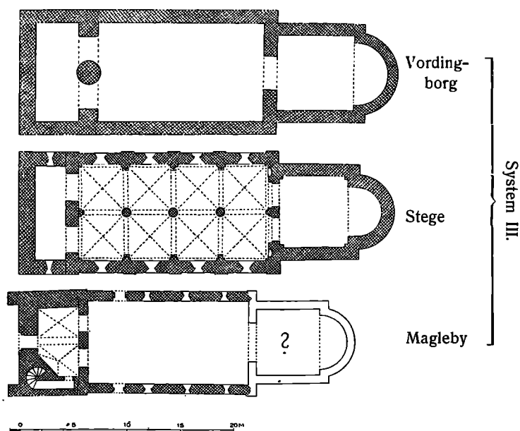
Fig. 11. Planer i 1:500 af de tre yngste Kirker med Tvillingtaarne.
