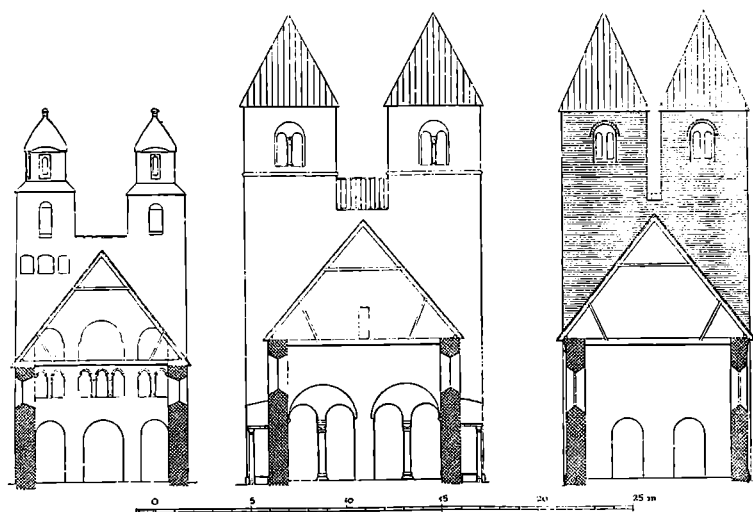
Fig. 12. Tveje Merløse, Färlöf og Magleby. Tværsnit, set mod Vest (1: 400).
