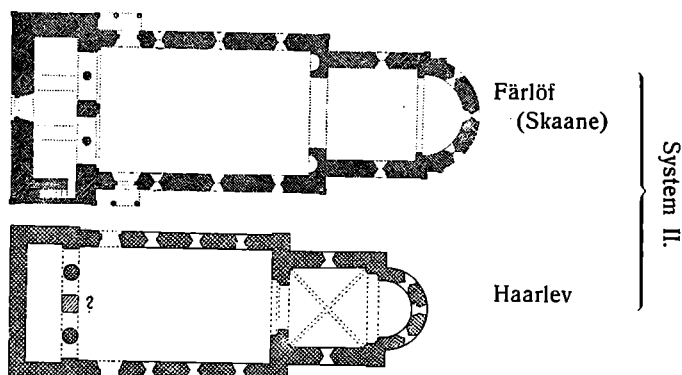
Fig. 10. Grundplaner i 1:500 af de to Kirkebygninger, ved hvilke Tredelingen er bevaret i Taarnrummet, men forladt ved Inddelingen af Skillevæggen mellem Taarne og Skib.
