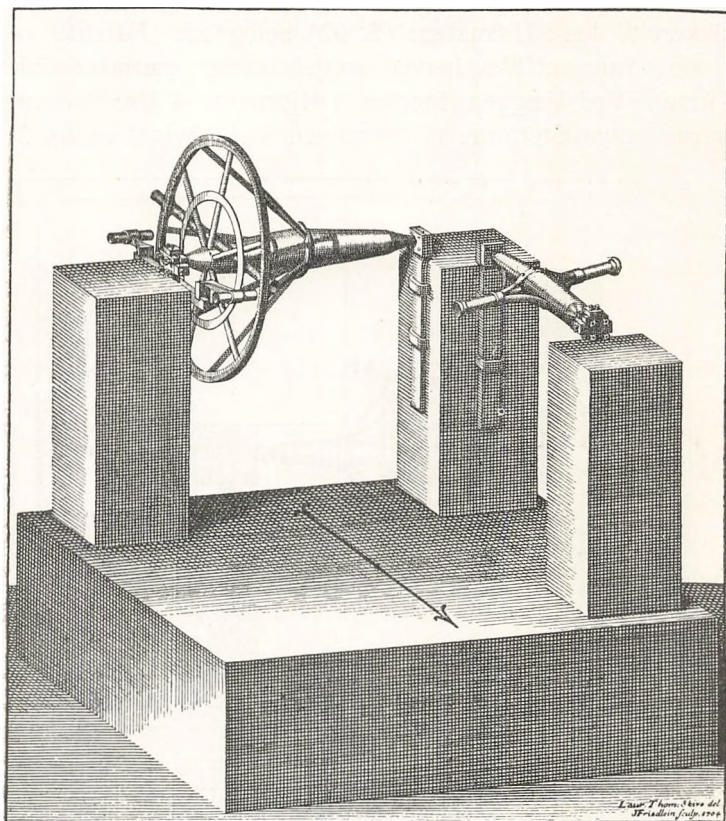
Fig. 4. Observatorium Tusculanum. Kikkertopstillingen.
