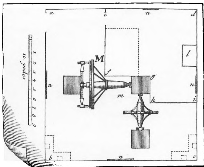
Fig. 3. Observatorium Tusculanum.
