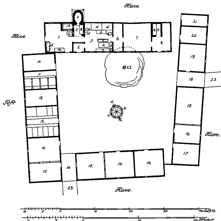
Fig. 5. Grundplan af en Gaard i Kløvested, Dalby Sogn. 1: 400.
