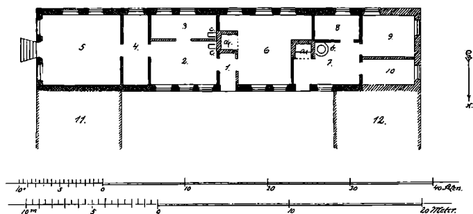
Fig 16. Grundplan af Vejlegaarden i Øverød, Søllerød Sogn. Opmaalt i 1926 og rekonstrueret af H. Zangenberg. 1:400.
