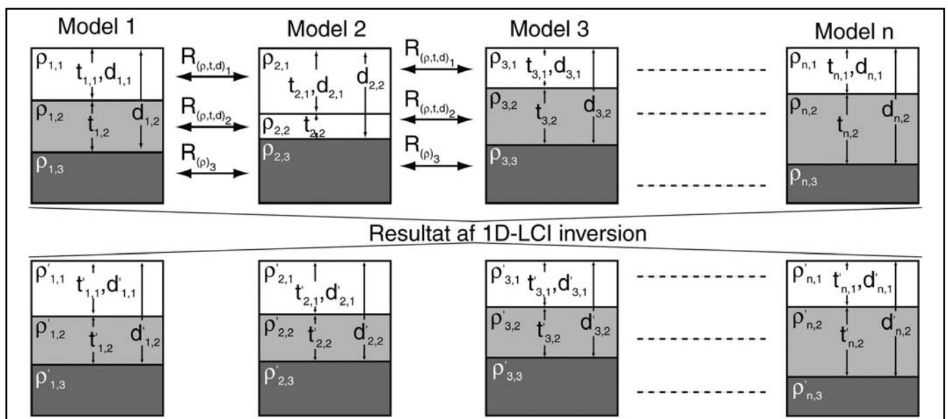
Principskitse af LCI-metoden. Øverst ses forskellige modeller, der via laterale bånd på modelparametrene bindes sammen. Dette resulterer i en udglatning, hvorved der opnås mere ens modeller. (Grafik: Lars H. Jacobsen)
