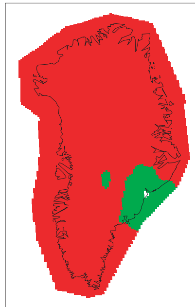
Her ses lokaliseringen af det glaciale jordskælv den 20. oktober 2000. Farver viser højden af bølgen i middel-seismogrammet for de forskellige test-epicentre. Hovedparten af test-epicentrene giver en bølge, som er lavere end tærskel-værdien (den røde farve). I ét område bliver bølgen høj nok til at registreres som et muligt jordskælv (det grønne område). Sandsynligheden for, at et jordskælv fandt sted, er størst i det hvide felt ved 68°N, 32°W. Kortet til venstre viser de områder, som samtlige de grønlandske glaciale skælv er fundet i. (Grafik: T. M. Jørgensen)
