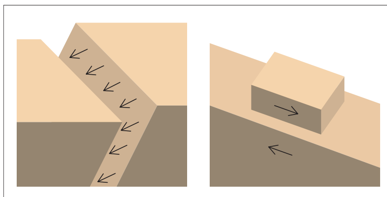
Venstre: Et normalt jordskælv beskrevet ved to blokke, som forskydes i forhold til hinanden. I dette tilfælde er den ene blok gledet skråt nedad uden at slippe kontakten med den anden blok, som har bevæget sig op. Højre: En jordskreds-model. En klump jord har løsrevet sig fra skrænten og glider/væltet nedad. Samtidig vil underlaget som modreaktion bevæge sig i modsat retning, altså opad og bagud. (Grafik: T. M. Jørgensen)
