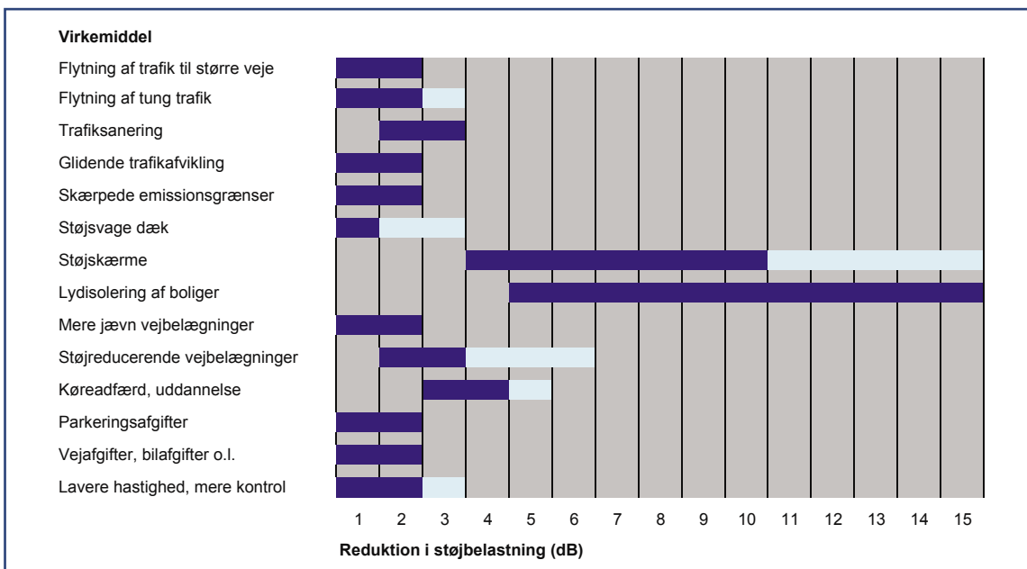
Figur 1. En oversigt over hvad man kan opnå af støjdæmpning er vist i figuren. Den mørke farve viser hvad der normalt kan forventes af støjdæmpning, mens den lyse farve viser hvad der i gunstige tilfælde kan opnås.
