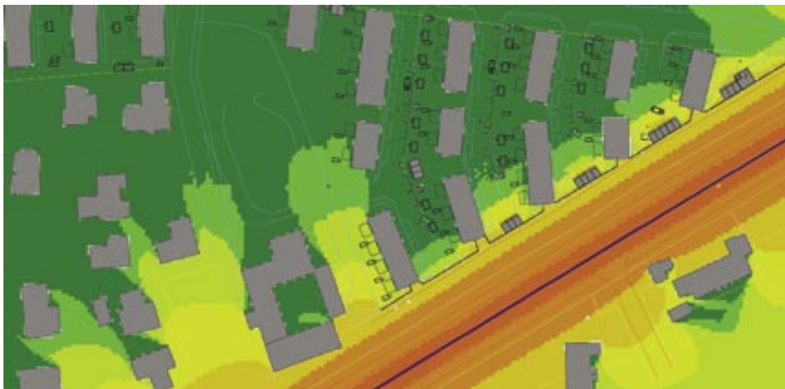
Figur 3: Støjudbredelse for et lokalplanområde beregnet ved hjælp af en GIS baseret støjmodel, som kombinerer støjberegningsmetode med digitale kort. Dette eksempel er udarbejdet med den tidligere nordiske beregningsmetode (NVB96)
