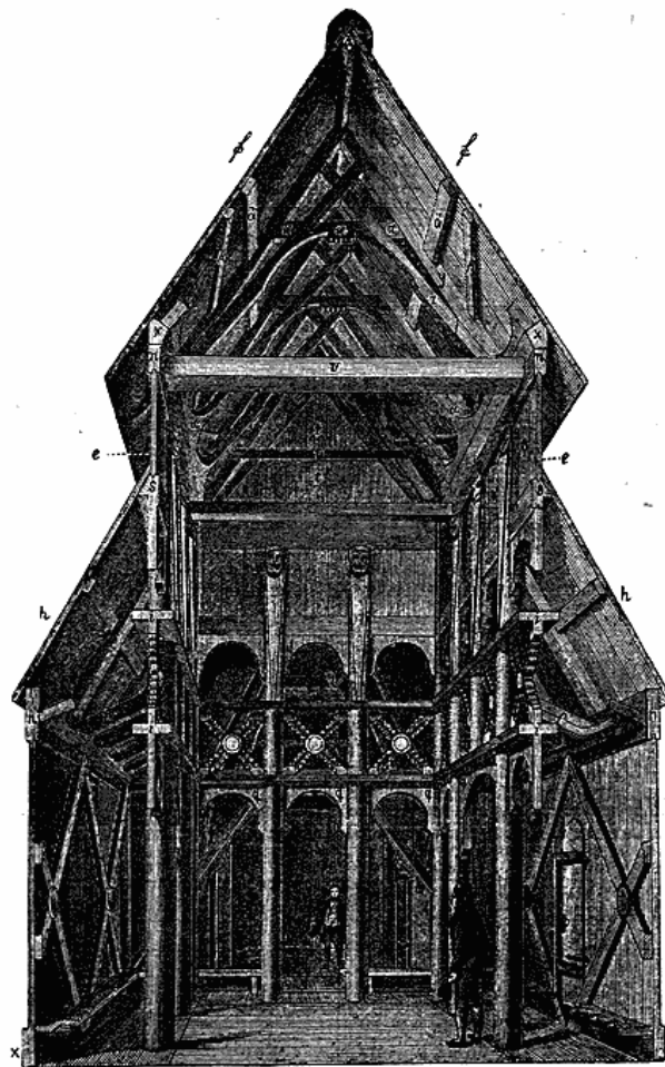
Fig. 5. Det indre af Borgund Kirke i Norge.
