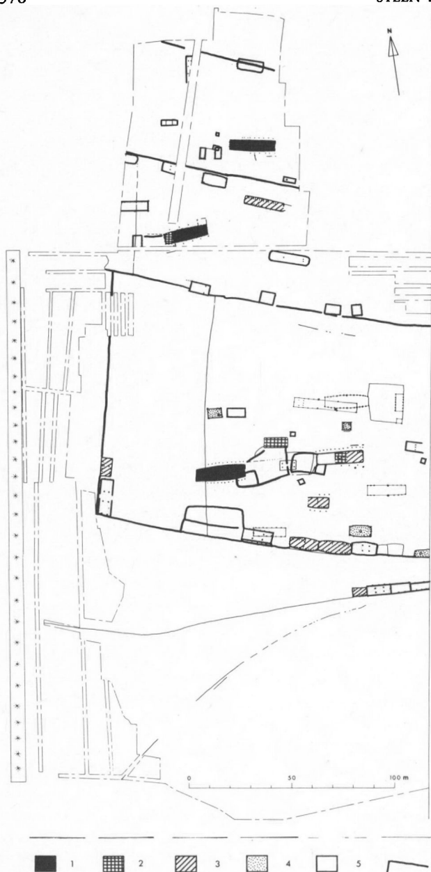
Fig. 15. Samlet plan over vikingetidsbebyggelsen. 1: Trelleborghuse. 2: Værksteder. 3: Stalde. 4: Mindre huse med ildsted. 5: Andre huse. 6: Hegn.
