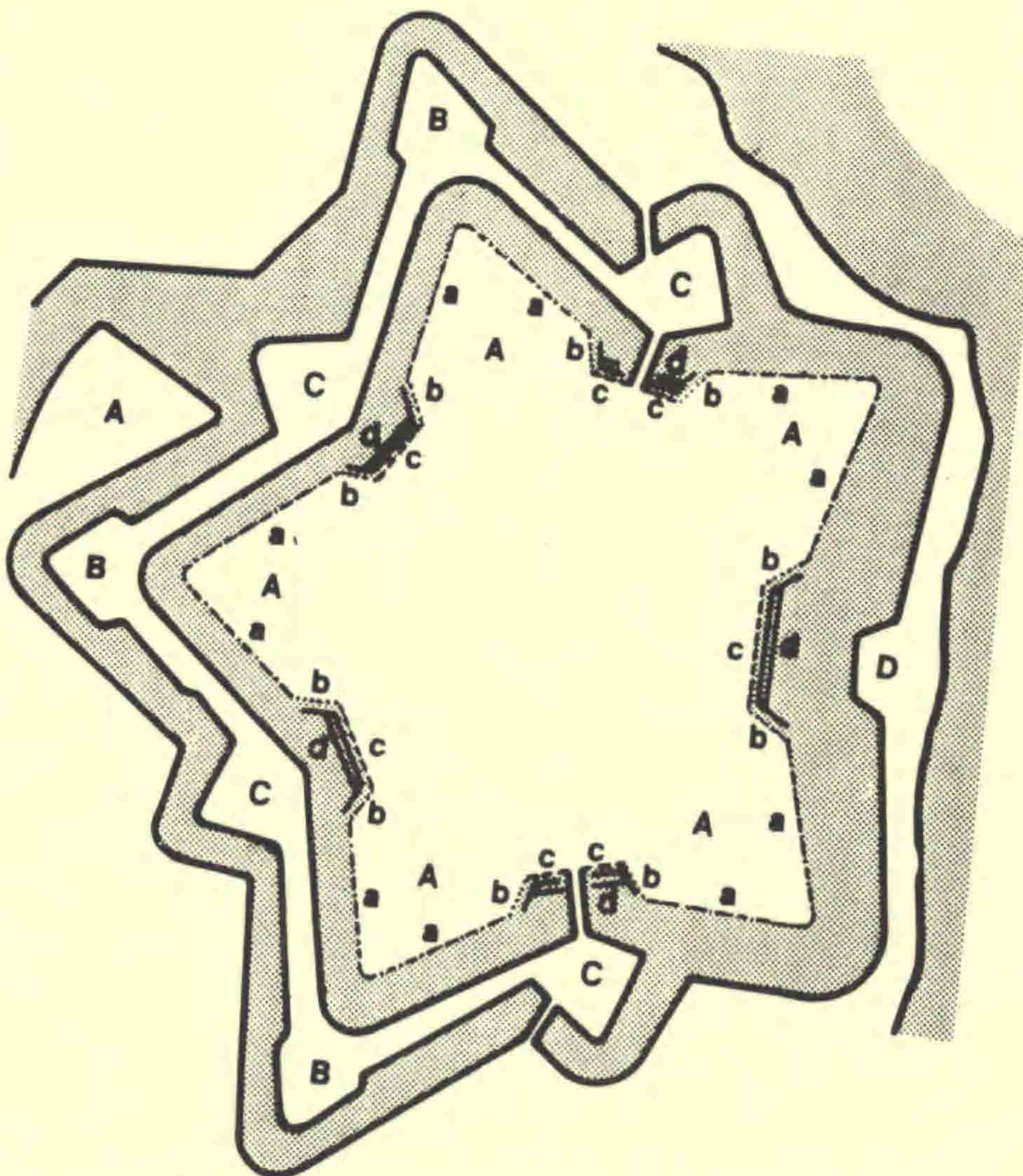
Fig. 4 De fortifikationstekniske betegnelser for voldanlæggets enkelte elementer (omtegnet efter figur side 16 hos Herluf Krabbe: Kastellet gennem 300 år. Martins Forlag 1964).
