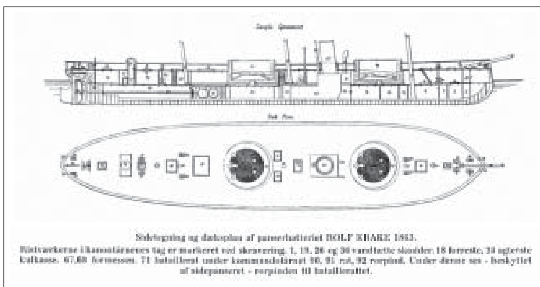
Rolf Krake. Sidetegning og dæksplan. (Steensen (1968), p. 210)
