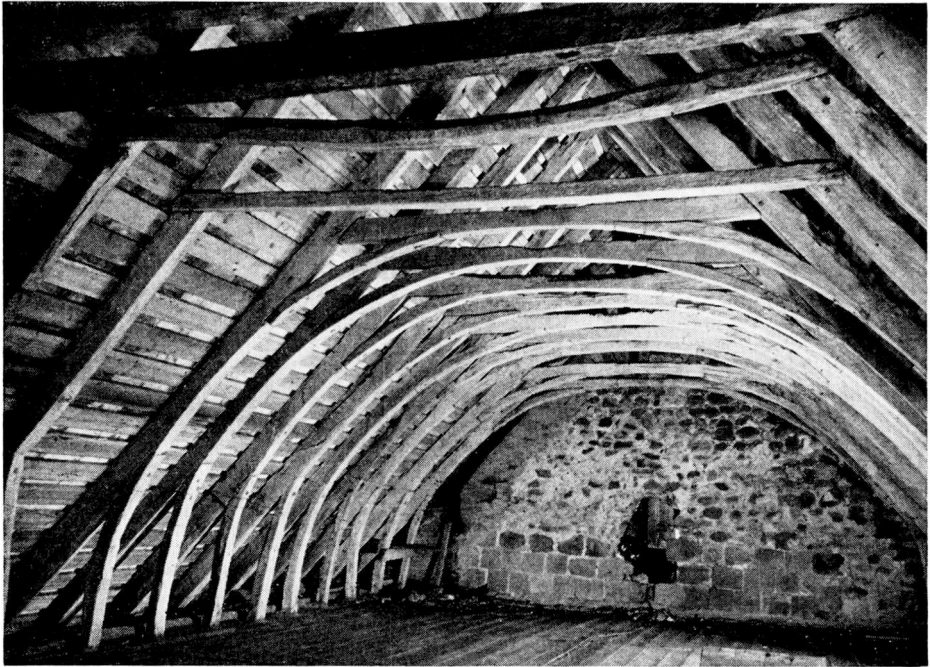
Fig. 1. Sædding kirke , Ringkøbing amt. Skibets tagværk set mod øst, med de buede spærfag over østenden og almindelige hanebånds-spærfag over vestenden. Det er en undtagelse, at skellet i stort set samtidige tagværker er så iøjenfaldende.
