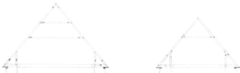
Fig. 2. Egvad kirke , Ringkøbing amt. Skibets tagværk med tømmernummerering, her udført som øksehugne stregnumre både i syd og nord, men en tværstreg udskiller den ene sides numre. Korets tagværk er nummereret med runer, og her er ligeledes benyttet en tværstreg som skille mellem nord- og sydsidens tømmer. I andre tagværker er numrene i nord og syd ofte udført med forskelligt værktøj.
