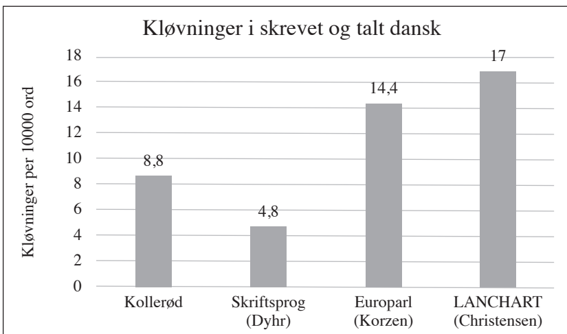
Figur 1. Antallet af kløvninger per 10.000 ord i denne undersøgelse og 3 andre danske undersøgelser
