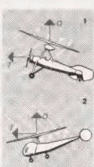
Helikopter. Den principielle forskel mellem autogyroen ① og helikopteren ②; O opdrift, T trækraft.
