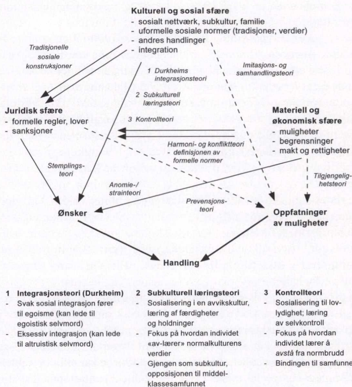
Figur 4.9 Samlet oversikt over ulike avviksteorier. Skjematisk fremstilling av teoriens hovedfokus. Heltrukne piler representerer faktorer som former individet, mens stiplede piler representerer faktorer som påvirker individets oppfatninger. Doppelpiler representerer faktorer som påvirker den juridiske sfæren. Tykke piler representerer aktørens handlingsvalg.
