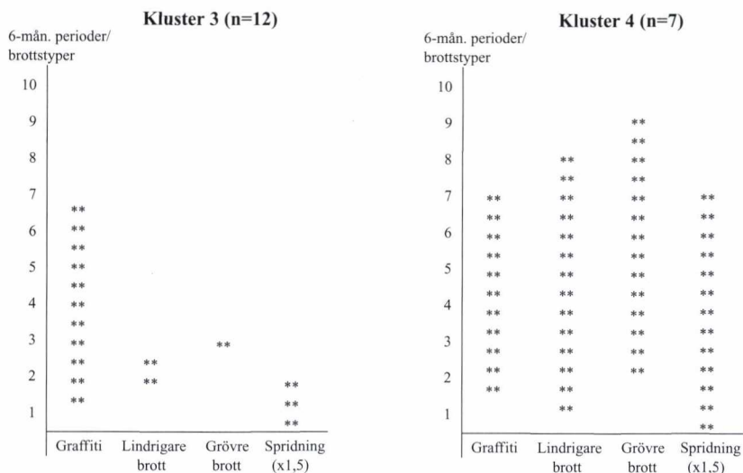
Figur 2. Medelvärdesprofiler för de slutgiltiga 'k-means' kluster 3 och 4.
