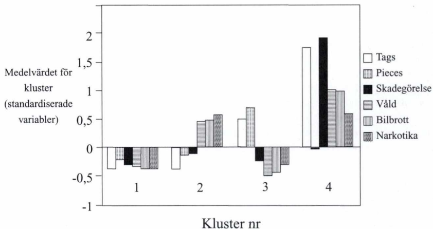
Figur 3. Medelvärdesklusterprofiler för antalet brott begåna i sex utvalda brottskategorier.
