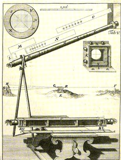
Figur 2. Tryk af Rømers gitterrør og amfioptr, som han beskrev og demonstrerede for Akademiets medlemmer [13], Tab. V).
