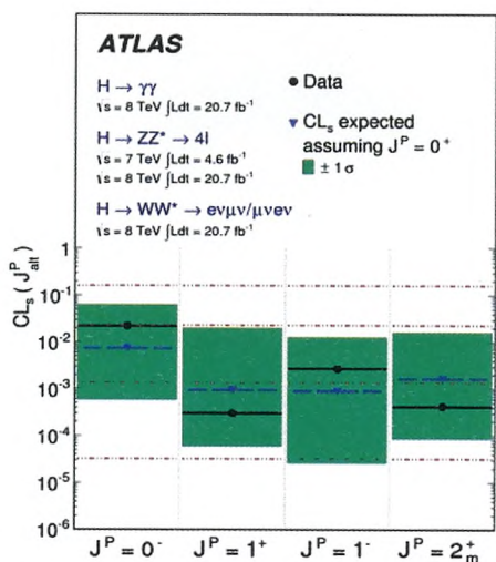
Figur 4. Øverst: Hvor stærkt den nye partikel vekselvirker med andre SM-partikler [2]. Nederst: Spin af den nye partikel. Eksklusion af andre muligheder end SM-forudsigelsen (spin 0 med paritet +) er nu 99,7 % sikker, bortset fra tilfældet med spin 0 og paritet -, hvor vi stadig har brug for mere data. "CL" på 2-aksen betyder "Confidence Level", der repræsenterer vores tillid (confidence) til, at udelukke hypotesen om en given kombination af spin og paritet ( J^P ) for partiklen. Hvis J^P = 1^+ har CL = 3 sigma, betyder det, at vi udelukker med 3 sigmas tillid (= 99,7 %) at Higgsen har J^P = 1^+ . Fra [3].
