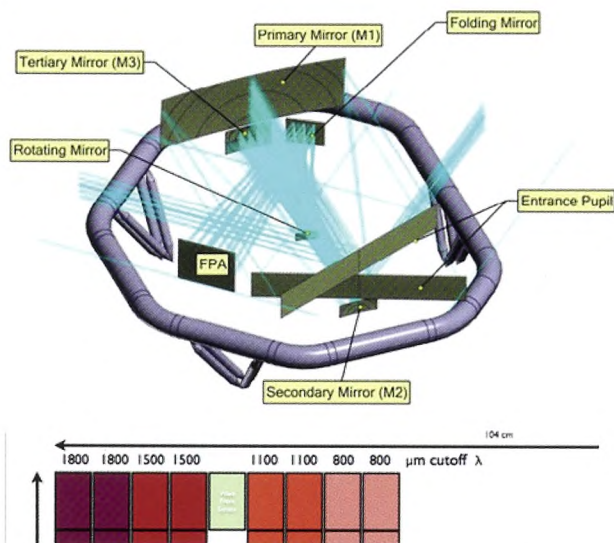
Figur 9. Gaia-efterfølger, kaldet GaiaNIR. Øverst: det optiske system, nederst: fokalanlæg, FPA, hvor kun den ene af syv rækker detektorer er vist. Disse detektorer skal udføre astrometri og samtidig fotometri ved fire bølgelængder mellem ca. 400 og 2000 nanometer.
