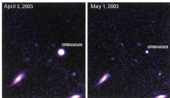
Figur 4. Lyset fra den eksplosion som forårsagede gammastrålingsglint GRB 030329. Astronomer fra Københavns Universitet deltog i disse observationer, som er udført med VLT [3]. (ESO Pressemeddelelse 16/03).
