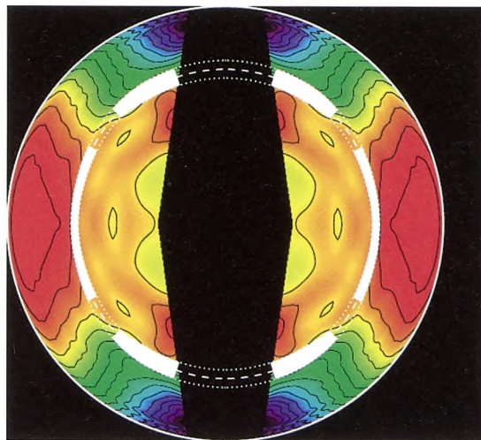
Figur 6. Rotationen i Solens indre, bestemt med helioseismologi. Farveskalaen markerer rotationsperioden, fra 25 døgne (rød) til 35 døgne (mørkeblå). I det sorte område omkring den lodrette rotationsakse er vi ikke i stand til at bestemme rotationshastigheden. De hvide områder markerer den såkaldte tachocline, hvor rotationshastigheden ændrer sig meget hurtigt mellem den ydre konvektionszone og det indre, hvor energien transporteres ved stråling.
