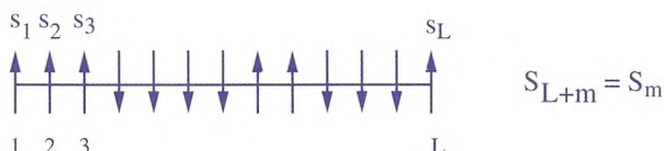
Figur 4. Heisenberg spinkæden med spin-1/2 variable på hvert gitterpunkt. En given spinkonfiguration svarer til en strengtilstand i den 10-dimensionale strengteori og et produkt af felter i den fire-dimensionale gaugeteori.
