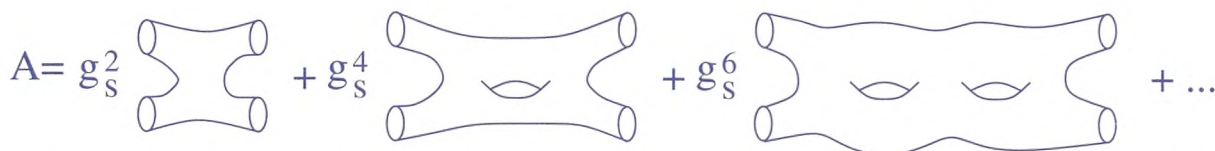
Figur 2. En spredningsamplitude for lukkede strenge kan skrives som en rækkeudvikling i g_s^2 . Denne rækkeudvikling kaldes for strengteoriens topologiske udvikling, idet den vægter strengenes verdensflader i henhold til deres topologi. Hvert håndtag på verdensfladen giver således anledning til en ekstra faktor g_s^2 . De tre verdensflader afbildet ovenfor har henholdsvis nul, et og to håndtag. Grænsen, g_s \rightarrow 0 svarer til frie, ikke vekselvirkende strenge.
