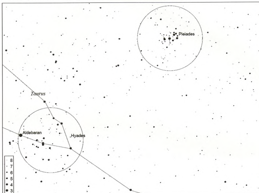
Figur 7. Kort, der viser stjernehoberne Hyaderne og Pleiaderne i Tyren . Kortet er 20° bredt. Det er fremstillet af Michael Quaade med XEphem programmet.
